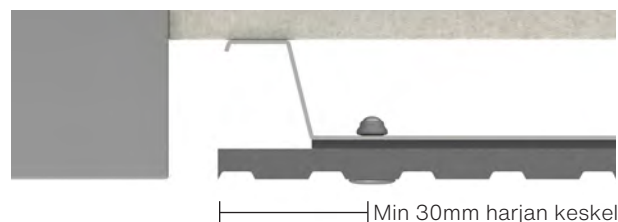
Kuva 4. Mittaan sahatun Swisspearl Patina Inline -levyn asennus
