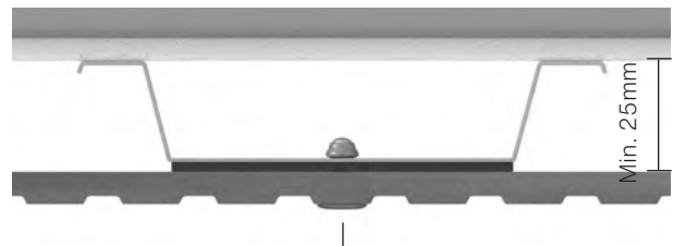
Kuva 1. Swisspearl Patina Inline -levyn asennus profiiliin liitoksen takana
