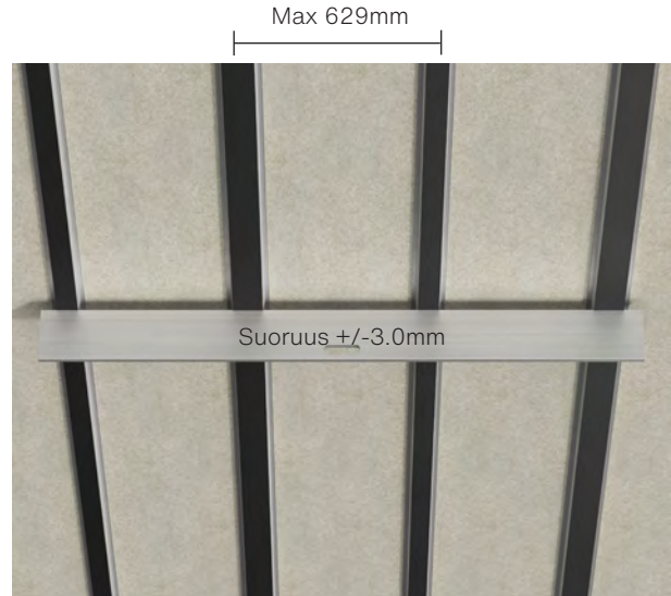
Alusrakenteen suoruuus
