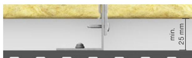
Rys. 2. Montaż Swisspearl Patina Inline na profilu „L”
