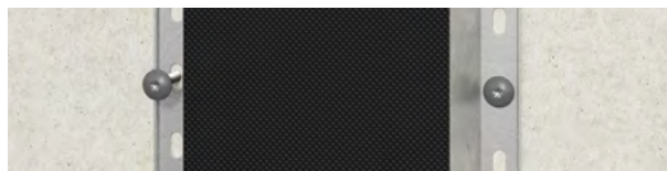
Rys. 2. Punkty przesuwne: profile Swisspearl „VFL” przykręca się za pomocą wkrętów umieszczonych pośrodku podłużnych otworów.
