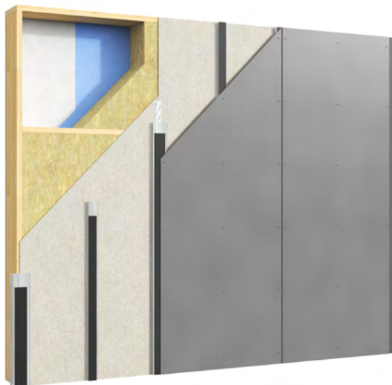
Lekka ściana z pionowymi profilami stalowymi „VFL”
