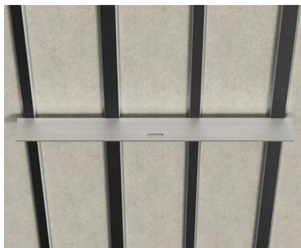
Prostoliniowość podkonstrukcji
