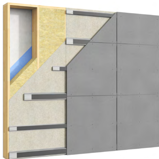
Lekka ściana z poziomymi stalowymi profilami „VFL”
