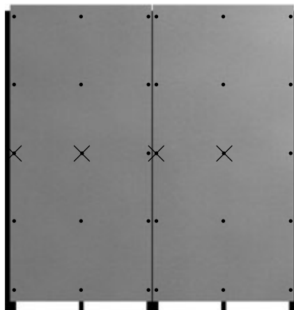
Przykład: Płyty montowane w układzie pionowym z jedną pośrednią łatą drewnianą
