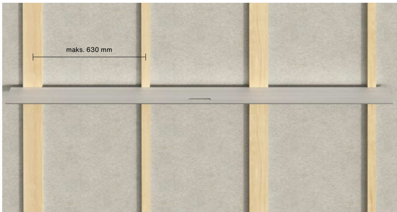
Prostoliniowość podkonstrukcji
