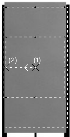
Ilustracja prawidłowej kolejności montażu wkrętów. Punkty stałe są oznaczone jako X
