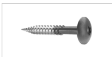
Wkręt fasadowy Swisspearl do drewna bez podkładki SCR-W 4,8×30/38/44 mm Stal nierdzewna A2 (Swisspearl Patina i Swisspearl Construction)
