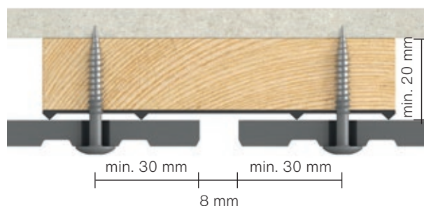
Rys. 1. Montaż Swisspearl Patina Inline na łącie wsporczej
