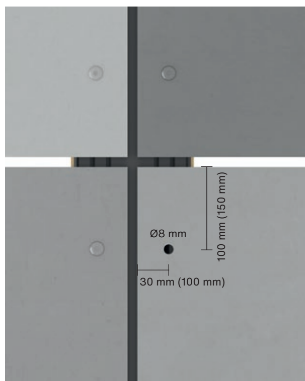
Przykład podkonstrukcji z układem pionowym – Swisspearl Cover, Swisspearl Solid i Swisspearl Transparent
