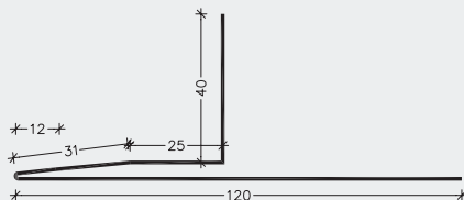
Swisspearl Lysningsprofil, lodret, Facadeskifer
