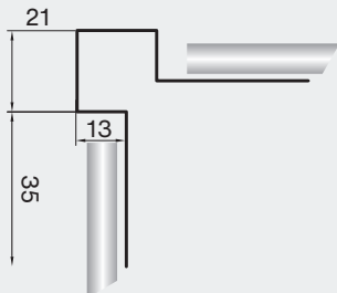
Swisspearl Indvendigt hjørne, kvadrat
