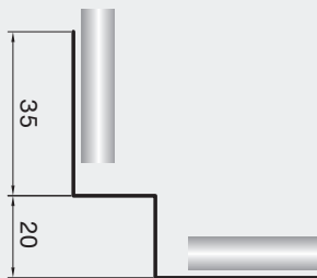
Swisspearl Indvendigt hjørne, kvadrat
