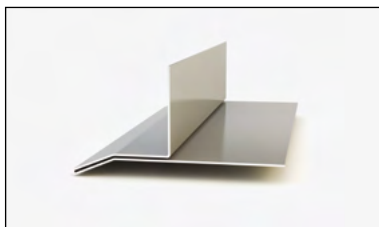
8. Swisspearl Lysningsprofil, vandret (stor) 40 x 50 x 40 mm farvet aluminiumsprofil til vandret afslutning over induer og døre.
