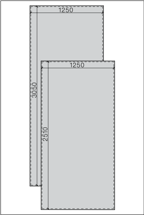
Wymiary użytkowe paneli o grubości 8 i 12 mm
