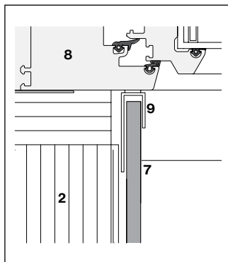
Lango angokraštis su metaliniu karkasu
