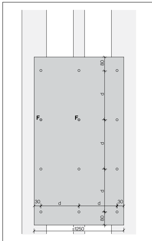
„Swisspearl Largo“ vertikali plokštė (stačia)
