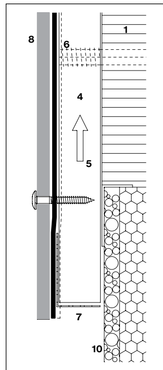
Mediniai vertikalusis tašai tvirtinami su distanciniais varžtais
