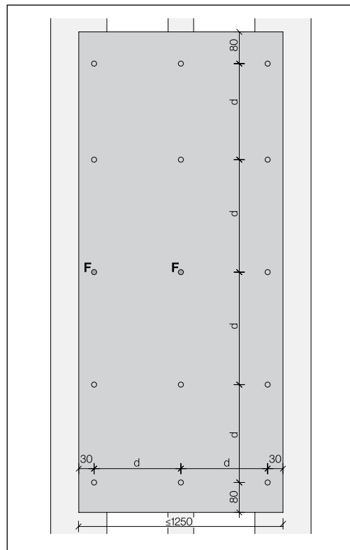
„Swisspearl Largo“ vertikali plokštė (stačia)
