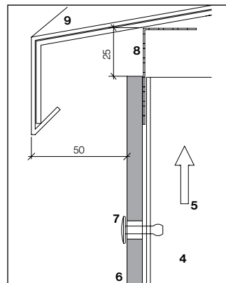
Palangės detalė
