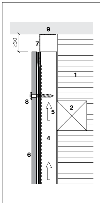
Fasado užbaigimo detalė po perdanga
