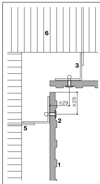
Exempel innerhörn
