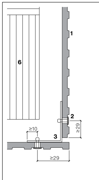
Exempel ytterhörn
