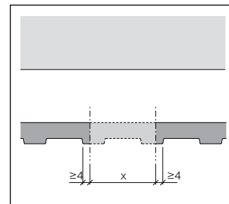
Gravial-bearbetning på byggplatsen
