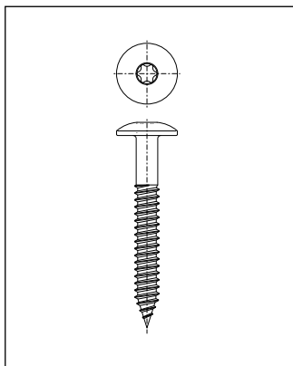
Swisspearl-skrue, rustfrit stål, rundt hoved Ø 12 mm, T20-drev.
