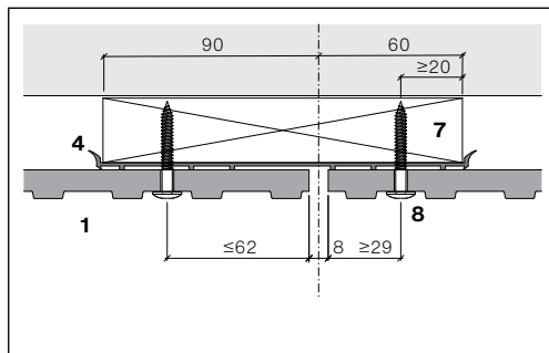
Trælægter 150 mm Individuelt Gravial-spor
