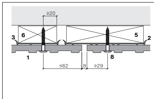
Trælægter 95 mm og 45 mm Individuelt Gravial-gitter
