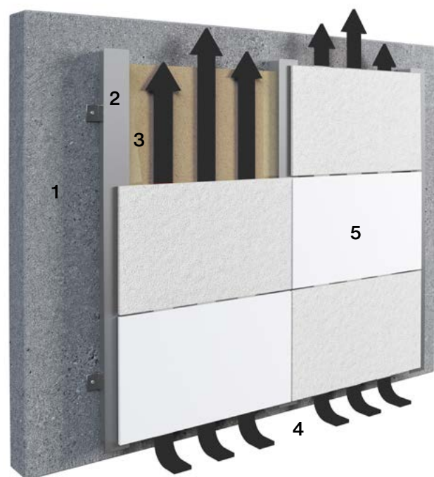
1 Tukirakenne, 2 Alusrakenne, 3 Lämmöneristys, 4 Tuuletusrako, 5 Swisspearl-kuitusementtilevyt
