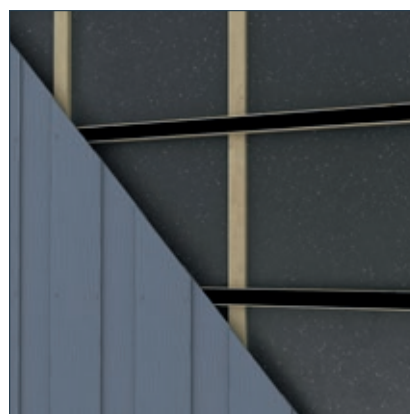
Verticale installatie op houten achterconstructie
