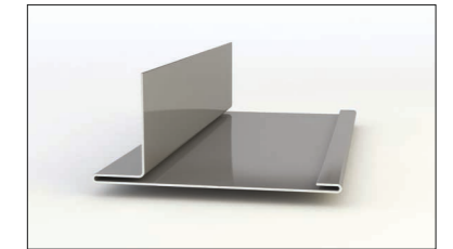
6. Swisspearl Lysningsprofil, lodret (stor) 40 x 21 x 79 mm farvet aluminiumsprofil til lodrette afslutninger omkring vinduer og døre.
