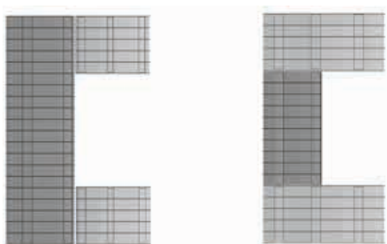
Esimerkkikuvat teräsrankojen liikuntasaumoista ikkuna-aukon ympärillä.
