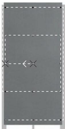
Illustrasjon av korrekt rekkefølge på naglemontering. X er faste punkter
