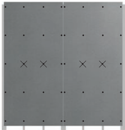
Eksempel: Vertikalt monterte plater med 2 mellomliggende aluminiumsprofiler.
