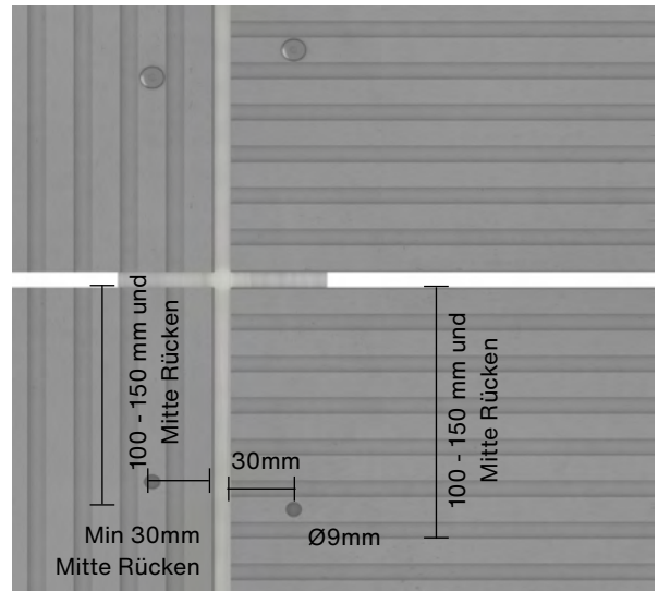
Abb. 3. Swisspearl Patina Inline NXT Randabstände
