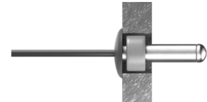
X: Festpunkt-Lochdurchmesser Ø 9 mm Verwenden Sie dazu die Swisspearl Festpunkthülse lt. Zulassung
