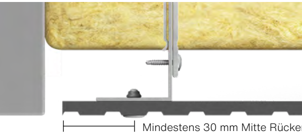
Abb. 4 Swisspearl Patina Inline NXT – ausgemittelte Befestigung auf dem Rücken
