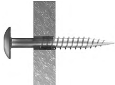
Swisspearl Patina NXT Design Line: X = Festpunkt: Lochdurchmesser Ø5 mm Gleitpunkt: Lochdurchmesser Ø8 mm
