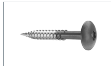
Swisspearl Fassadenschraube 4,8 x 44 mm V2A / V4A für sichtbare Befestigung auf Holz-UK. In allen Farbtönen erhältlich
