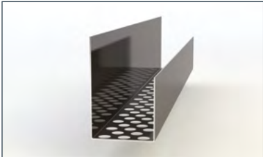
Swisspearl Hinterlüftetes Wandprofil 40 25 x 40 mm Horizontale Belüftung 1 mm Anfangs-Anschluss-Stahlprofil
