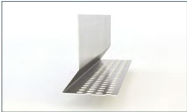
2. Swisspearl Planks Anfangs-Lüftungsprofil 25 x 48 mm Aluminium-Anfangsprofil für Planks
