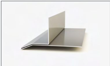
8. Swisspearl Horizontale Leiste groß 40 x 50 x 40 mm farbige Aluminiumleiste für Fenster- und Türeinfassungen
