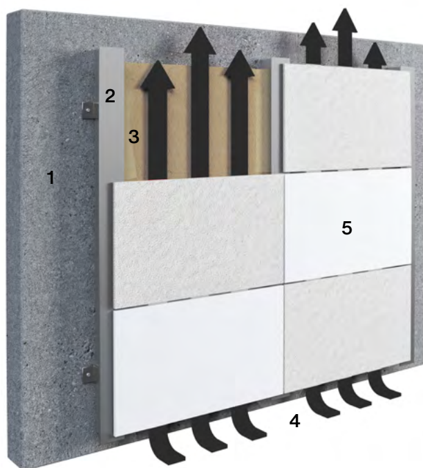
1 kandekonstruktsioon, 2 alusstruktsioon, 3 soojusisolatsioon, 4 tuulutusvahe, 5 Swisspearli kiudtsementplaadid
