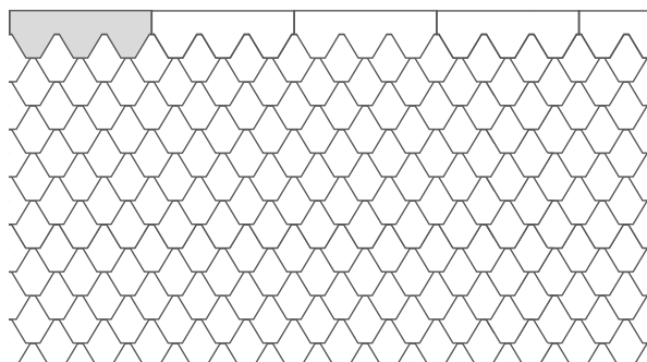
Kärjekujuline 600 x 200 x 4 mm (3 x 200 x 200 x 4 mm)
