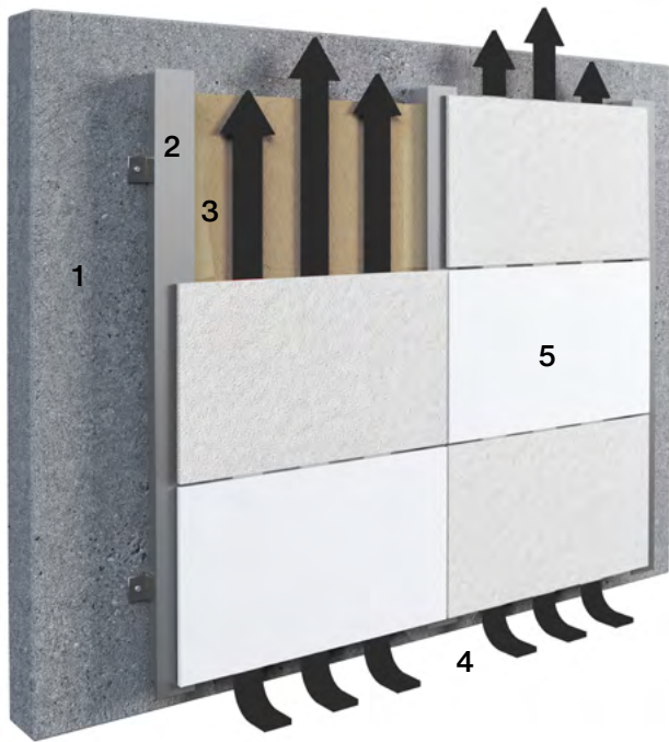
1 kandekonstruktsioon, 2 alusstruktuur, 3 soojusisolatsioon, 4 tuulutusvahe, 5 Swisspearli kiudtsementplaadid
