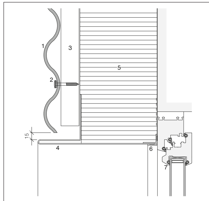
Verlegung horizontal
