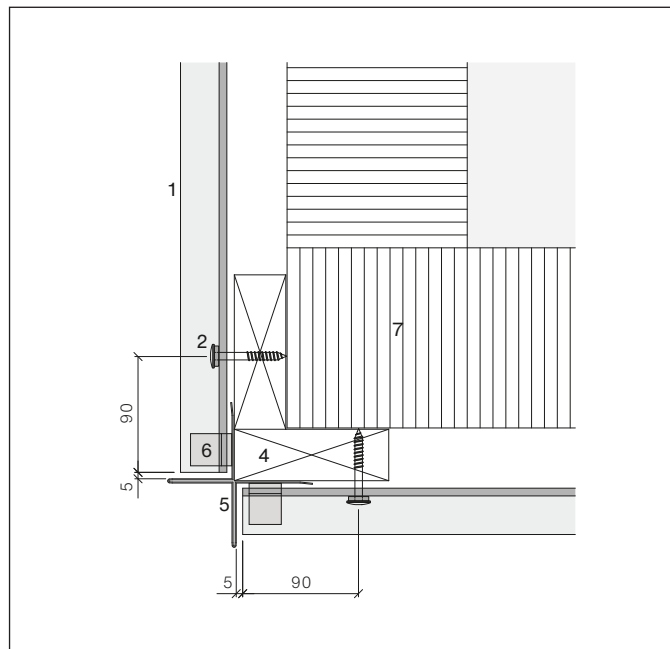
Verlegung horizontal
