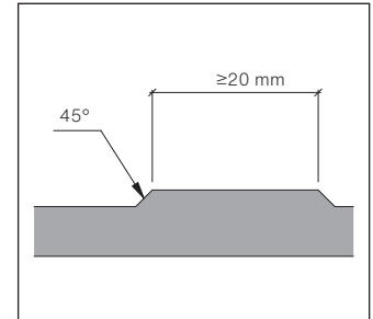
20 mm Minimaler Abstand von Ausfräsung zu Ausfräsung oder zum Plattenrand
