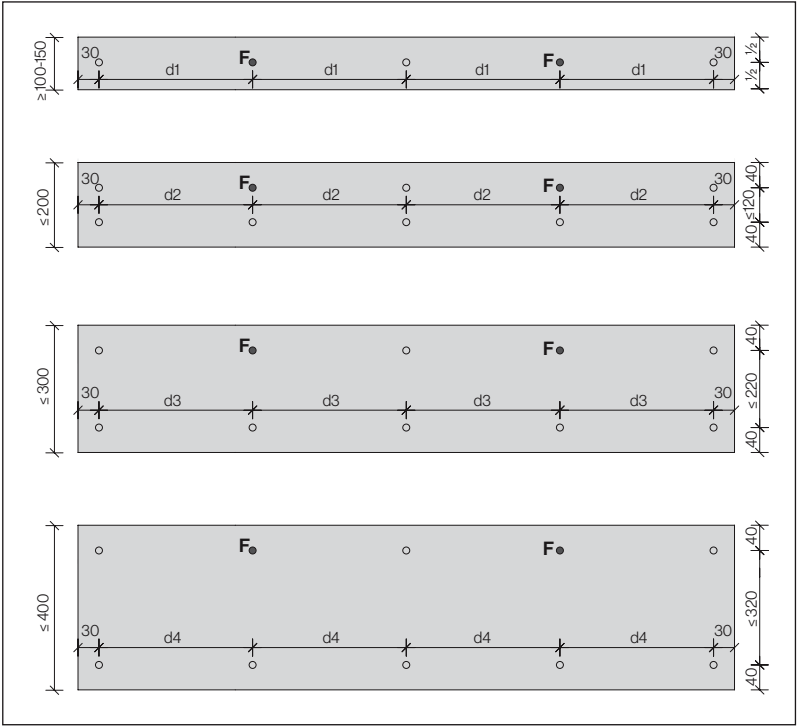
Festpunktanordnung bei einer horizontalen Largo-Streifenverlegung.
