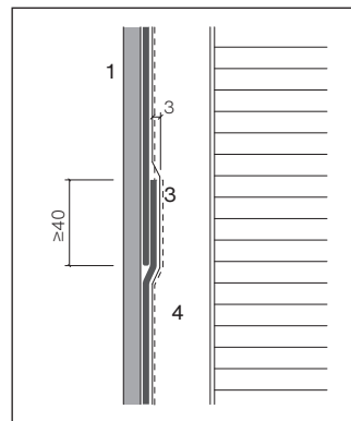
Stossfugen mit EPDM-Bändern
