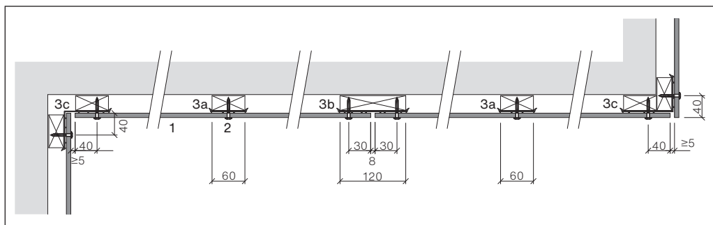
Horizontalschnitt mit Traglatten
