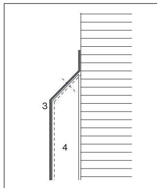
Nicht durchgehende Latten
