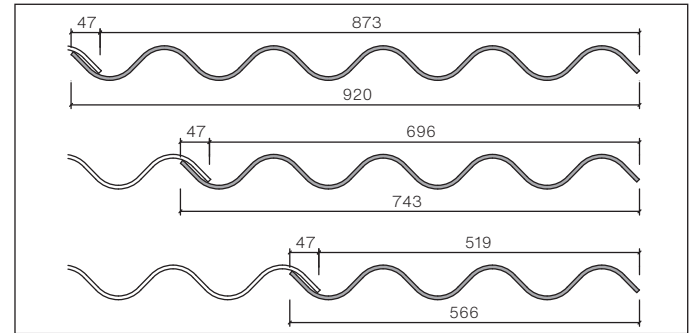
Ortplatte rechts
