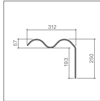
Ortabschluss R
