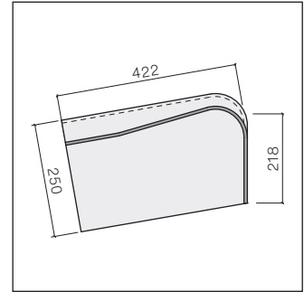
Pultfirstkappen-Abschluss 80°
