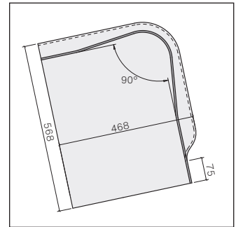
Shedfirstkappen-Abschluss 90°
