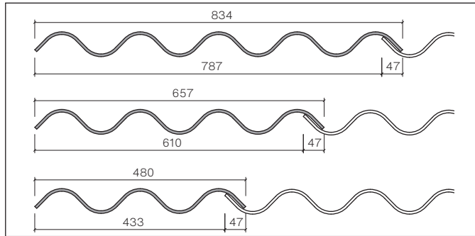
Ortplatte links
