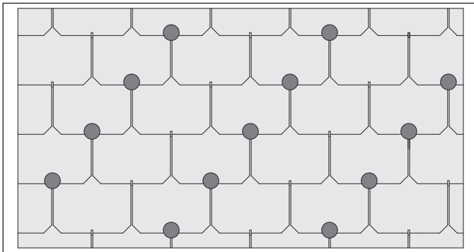
Bezugshöhe bis 700-1100 m, Dachneigung bis 25° 5.1 Stück/m 2
