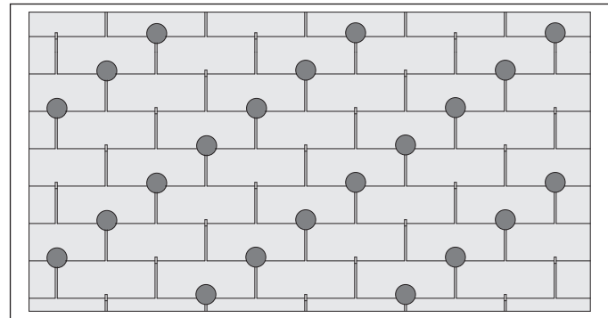
Bezugshöhe bis 700-1100 m, Dachneigung bis 26-45° 8.7 Stück/m 2
