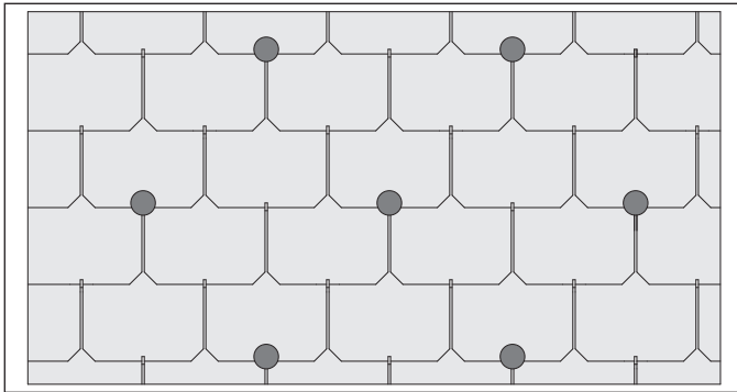
Bezugshöhe bis 700 m, Dachneigung bis 25° 2.6 Stück/m 2
