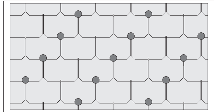
Bezugshöhe bis 700 m, Dachneigung bis 26-45° 5.1 Stück/m 2
