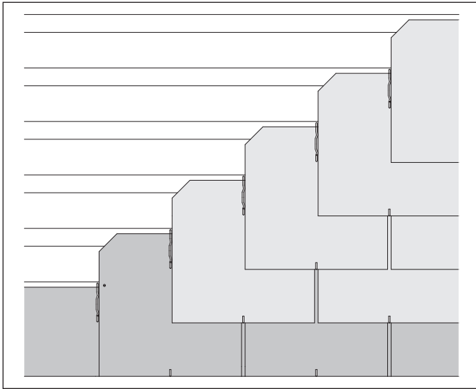
Beispiel Randbefestigung Traufe, Doppeldeckung
