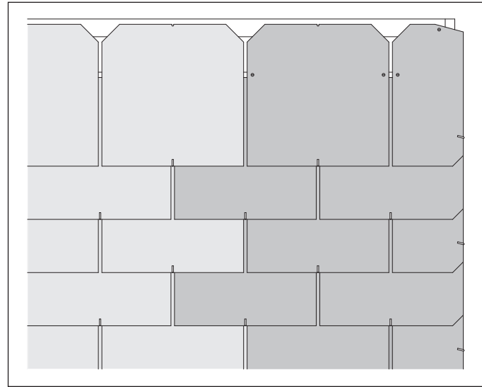
Beispiel Randbefestigung Ort, Doppeldeckung
