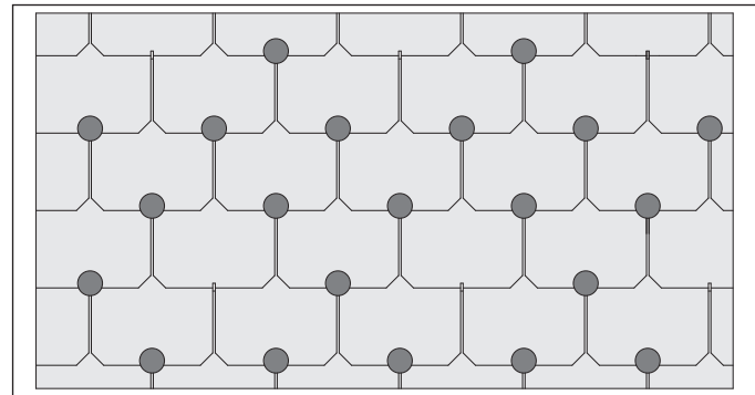
Bezugshöhe bis 700-1100 m, Dachneigung bis 26-45° 8.1 Stück/m 2
