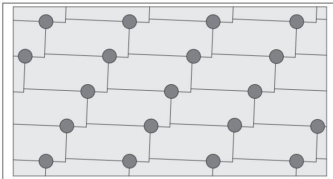
Verlegeschema 720×400 mm
