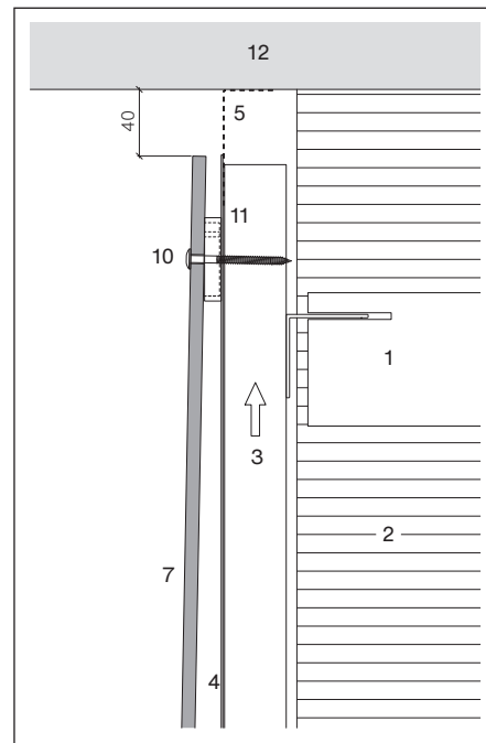
Anschluss mit Ergänzungsplatten, sichtbar befestigt
