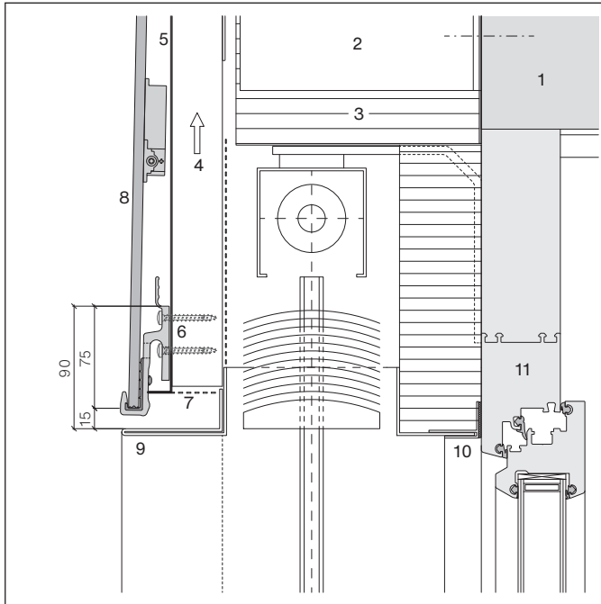
Fensterzarge Vertikalschnitt, Sturz mit Lamellenstoren
