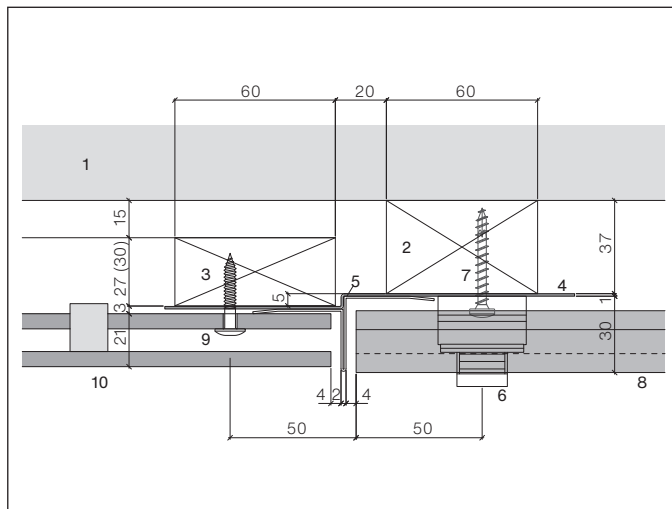
Horizontalschnitt, Fassadenanschluss zu Clinar Clip 6 mm
