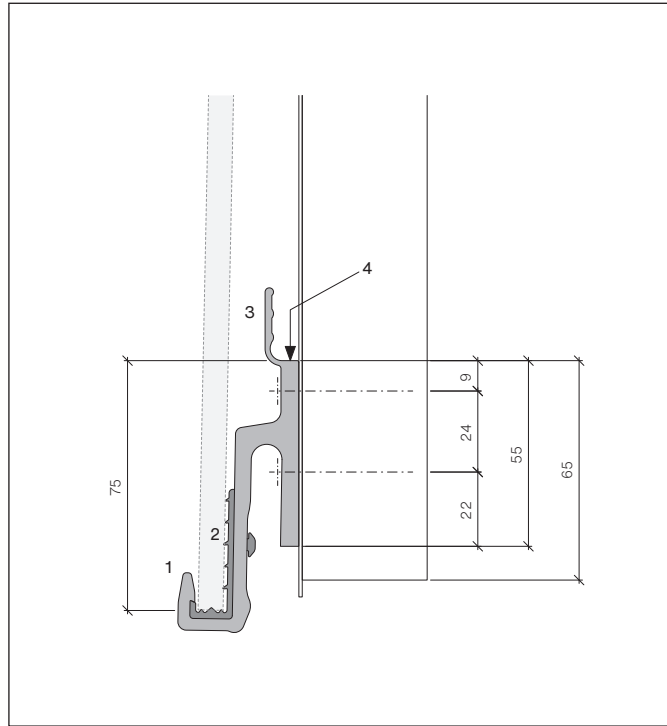
Befestigung mit 2 Schrauben, 5.0×40 mm pro Modulhalter An- fänger
