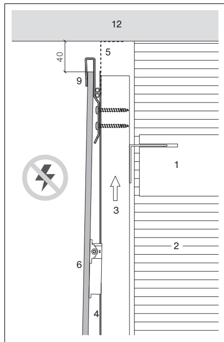
Anschluss mit PV-Modul bei der Zwischenauflage
