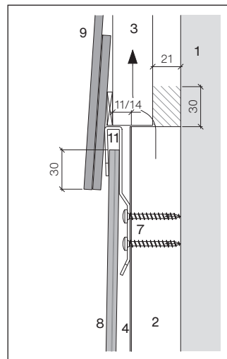
Vertikalschnitt, Fassadenanschluss zu Clinar Stülpedeckung 6 mm
