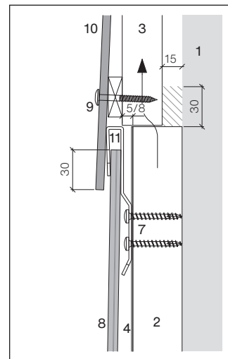
Vertikalschnitt, Fassadenanschluss zu Clinar Clip 6 mm
