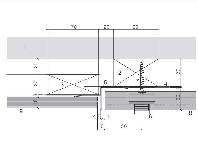
Horizontalschnitt, Fassadenanschluss zu Clinar Stülpedeckung 6 mm
