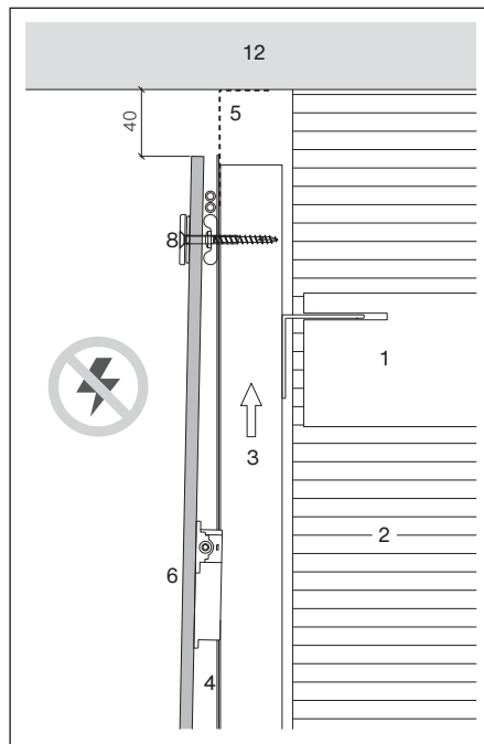
Anschluss mit PV-Modul bei der Vertikal- fuge
