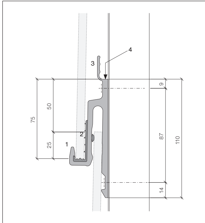
Befestigung mit 2 Schrauben, 5.0×40 mm pro Modulhalter
