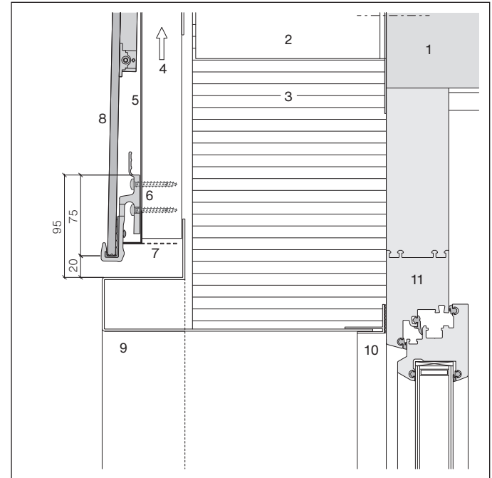
Fensterzarge Vertikalschnitt, Sturz geschlossen
