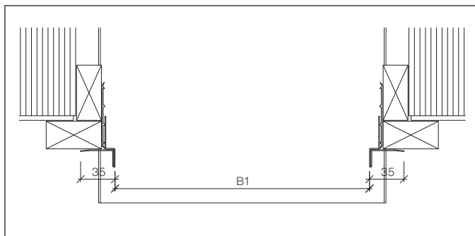
5. Sturzprofilbreite bestimmen
