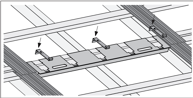
Modulhalter einlegen.
