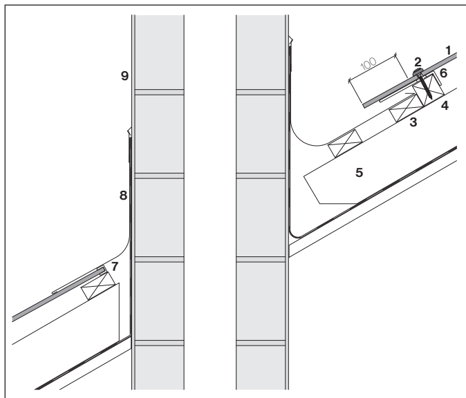
Kaminanschluss, Vertikalschnitt
