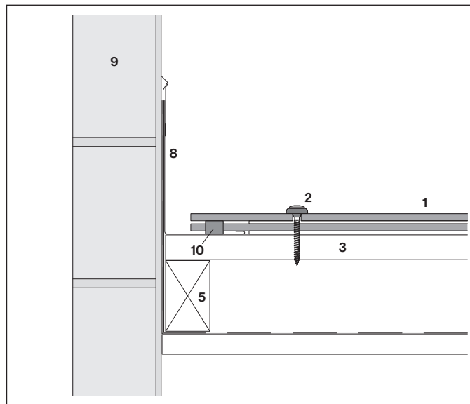
Kaminanschluss, Horizontalschnitt
