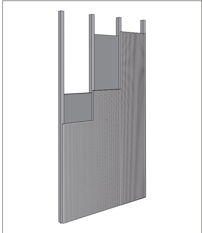
Beispiel Wandaufbau ohne Hohlraum
