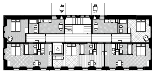
2. Obergeschoss
