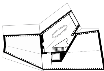
Obergeschoss
