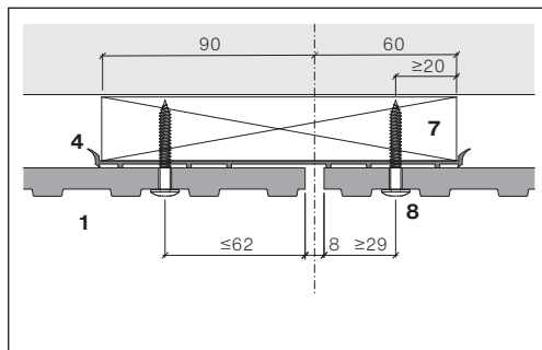
Koka brūsi, 150 mm Dalīts (deformācijas šuves) Gravial izkārtojums
