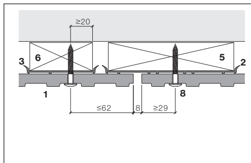
Koka brūsi, 120 mm un 60 mm Dalīts (deformācijas šuves) Gravial izkārtojums
