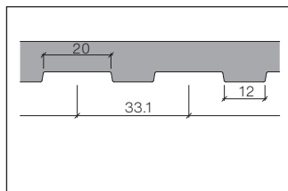
Detalizācija: Grival gravējuma izkārtojums
