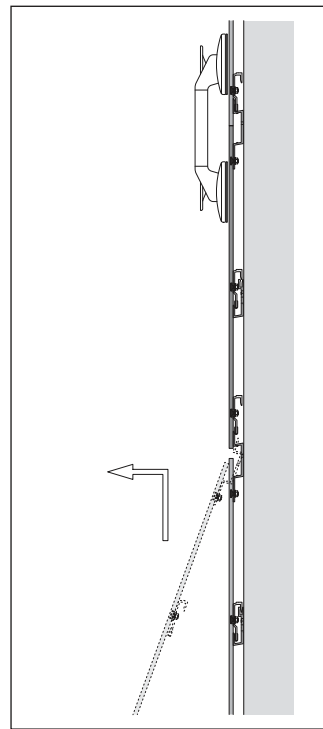
Paceliet un atāķējiet bojāto plāksni.
