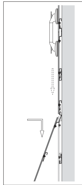
Piestipriniet jaunu plāksni nomaināmā vietā, nostipriniet to un atkārtoti nostipriniet augšējo plāksni. Sastatņu enkuriem procedūra ir tāda pati.
