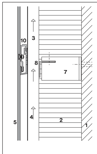
Koka/metāla apakškonstrukcija, termiskajam tiltam optimizēta apakškonstrukcija
