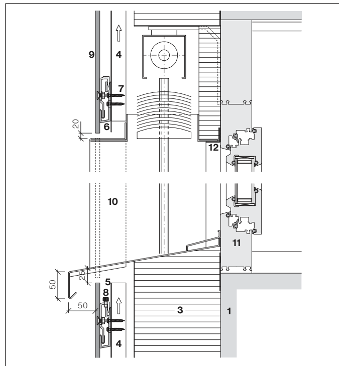
Loga aila, vertikāls griezumš
