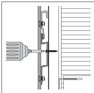
Koka karkasa gadījumā atskrūvējiet skrūves
