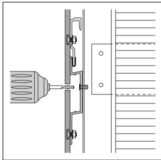
Metāla karkasa gadījumā izurbiet kniedes
