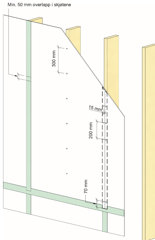
Fig. 1 Cembrit Windstopper montert på yttervegg med trestendere med tape over alle plateskjøtene.
