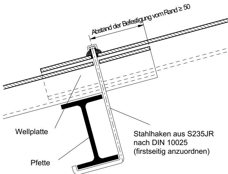
Bild 4.1: Anordnung der Befestigung mit Stahlhaken auf Stahl-Unterkonstruktionen
