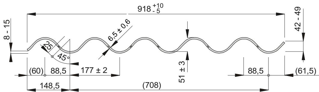
Bild 1.1: Faserzementwellplatte "Cembrit W177-5,5 RC" (Profil 5) mit PP-Bändern; Querschnittsabmessungen und Lage der PP-Bänder
