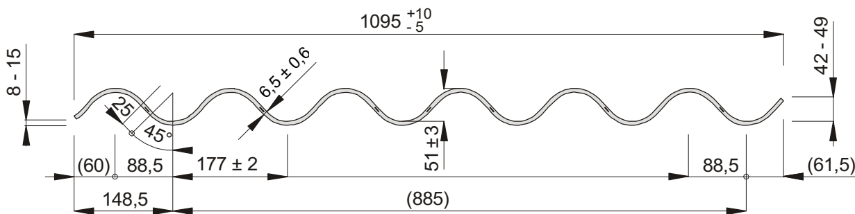
Bild 1.2: Faserzementwellplatte "Cembrit W177-6,5 RC" (Profil 6) mit PP-Bändern; Querschnittsabmessungen und Lage der PP-Bänder
