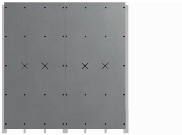
Fig. 2 Eksempel: Lodret monterede plader med to mellemliggende stålprofiler
