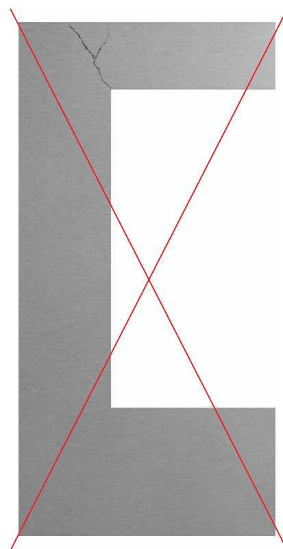
Forkert montering af facadeplader ved vinduer, døre og øvrige facadegennembrydninger.
