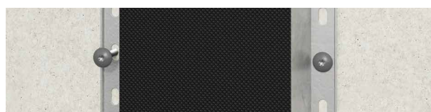
Fig. 3 I glidepunkterne monteres Swisspearl Montageprofiler med to skruer over for hinanden for at undgå forvridninger i stålet.
