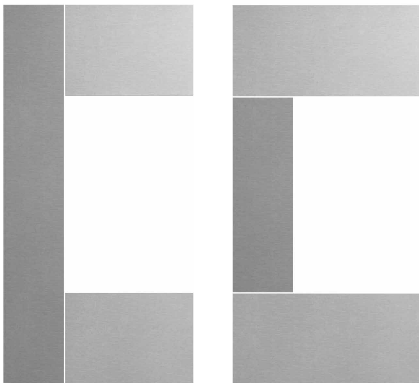
Korrekt montering af Swisspearl Facadeplader ved vinduer, døre og andre facadegennembrydninger.
