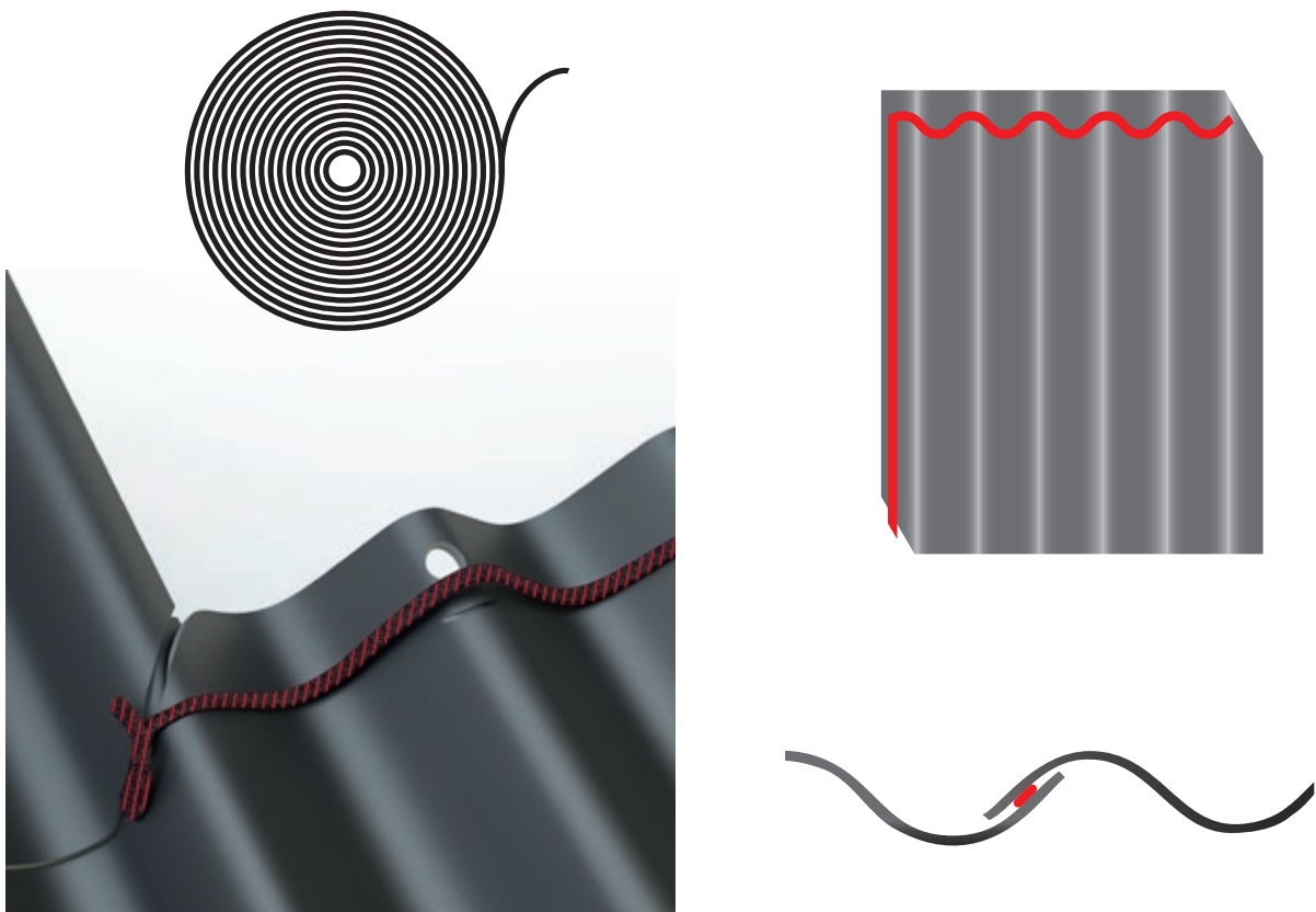
Fig 7.0 - Voorbeeld afdichtingsband
