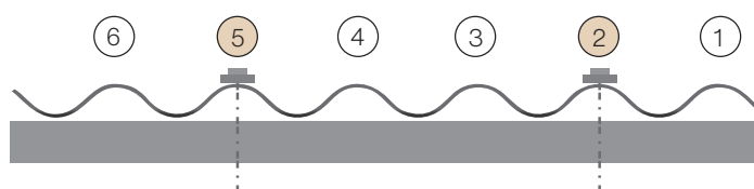
Fig 6.0 - Positie boutgaten
