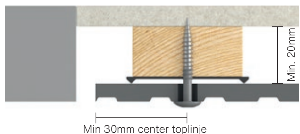
Figur 4. Skruelacering på tildannede plader ifm. Patina Inline.
