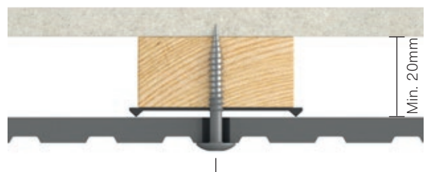
Figur 2. Montering af Patina Inline på bagvedliggende forskalling.
