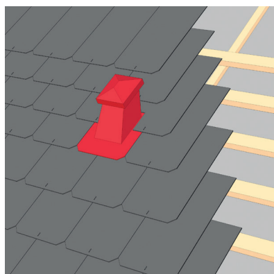
Swisspearl 30x60 skiferplader over hætten tilskæres som vist.
