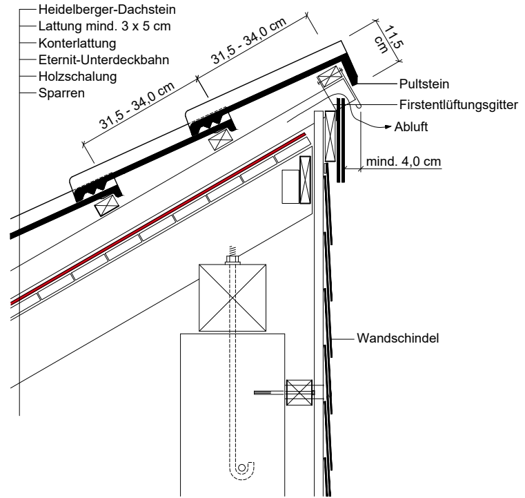
Halbfirst mit Heidelberg-Pultstein
