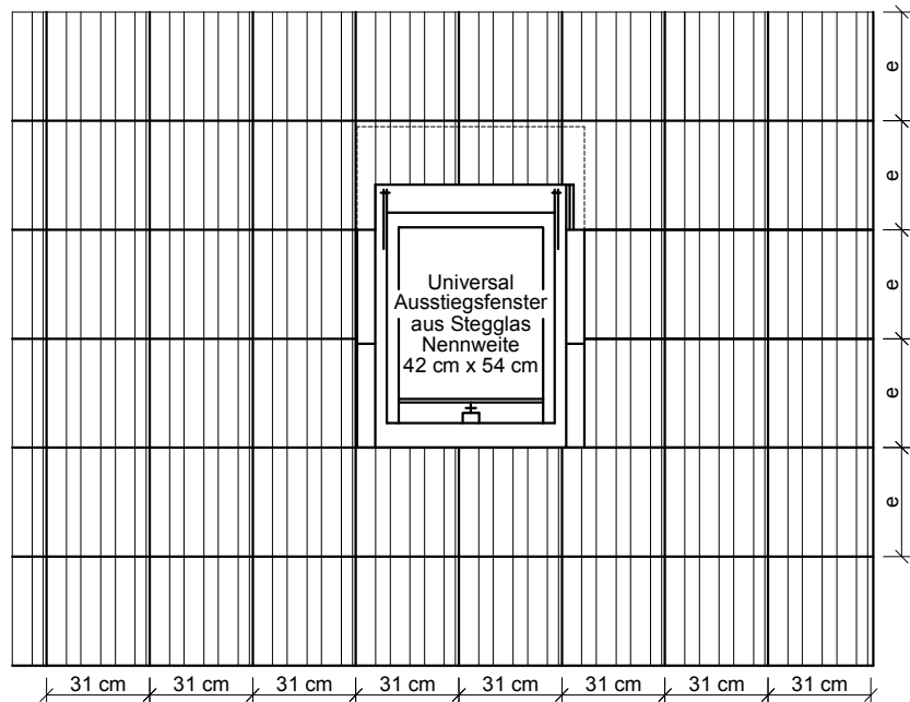
Ausstiegsfenster aus Stegglas
