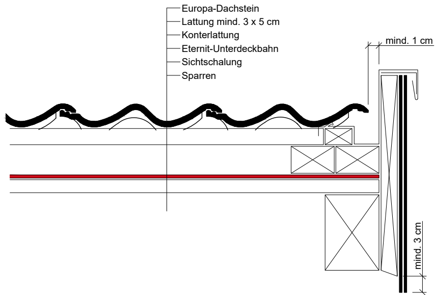
Ortgang mit Blech
