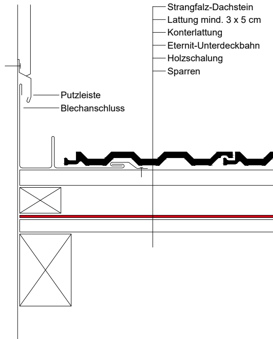
Wandanschluss - seitlich
