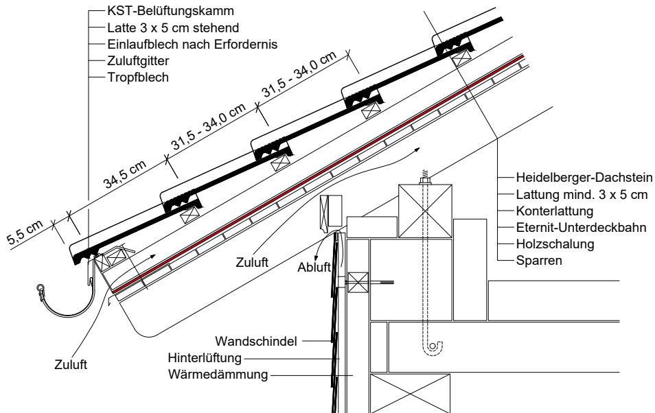
Traufe bei hohen Schneelasten
