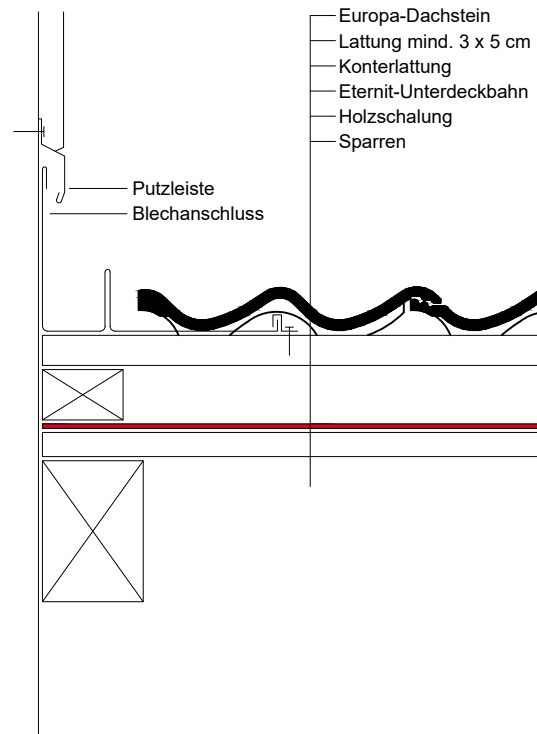
Wandanschluss - seitlich
