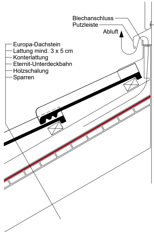
Wandanschluss - Firstseitig
