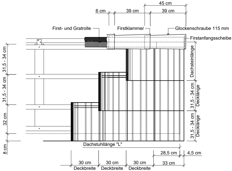
Deckstruktur
