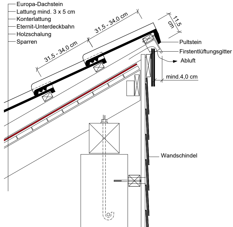
Halbfirst mit Europa-Pultstein
