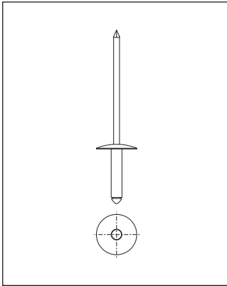
Rivet pour façade, tête de Ø15 mm, 4,0x18-K15
