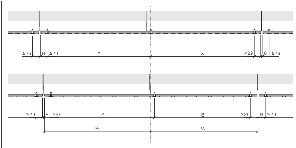
Découpe Gravail sur chantier
