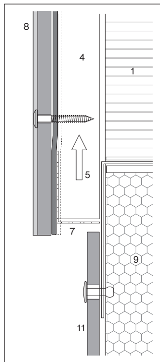
Ossature bois/métal
