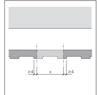
Découpe Gravail sur chantier
