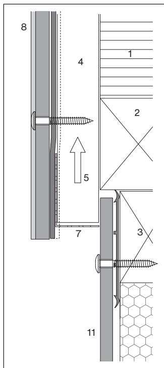
Ossature bois/bois
