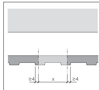
Découpe Gravier sur chantier
