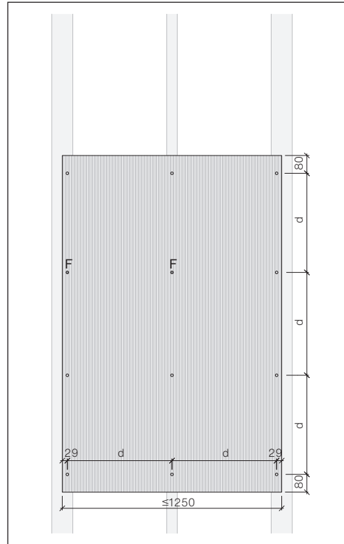
Largo Gravial disposition verticale
