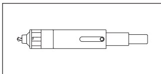
Guide de centrage 9541-2 avec foret Ø4.1 mm intégré:
