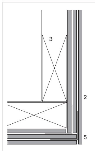
Ardoises coïncidentes Lattage vertical 27×70 mm
