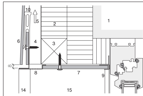
Linéau avec plaque Largo
