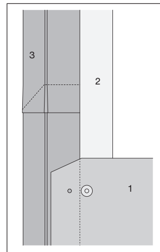
Angle extérieur
