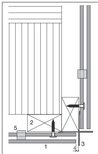
Profilé d'angle cruciforme, âme 24 mm
