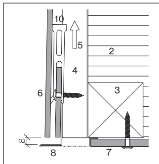
Linéau avec profilé de finition
