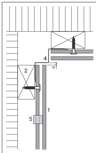
Profilé d'angle intérieur, âme 24 mm
