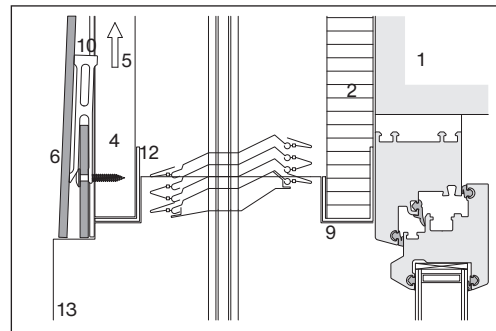
Linéau avec store ou volet roulant
