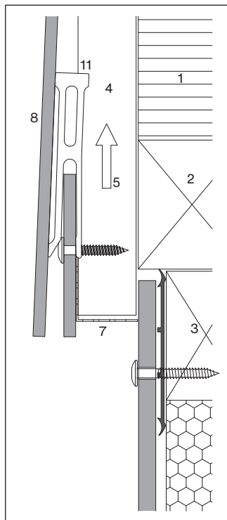
Ossature bois/bois
