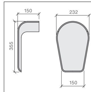
About de faîtière d'aération
