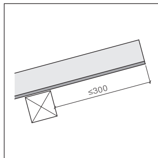
Débordement max. au faîte pour altitude de référence jusqu'à 1000 m
