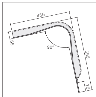
Faîtière shed 90°
