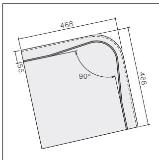
About de faîtière angulaire 90°
