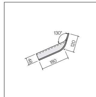
Raccord de faîtage
