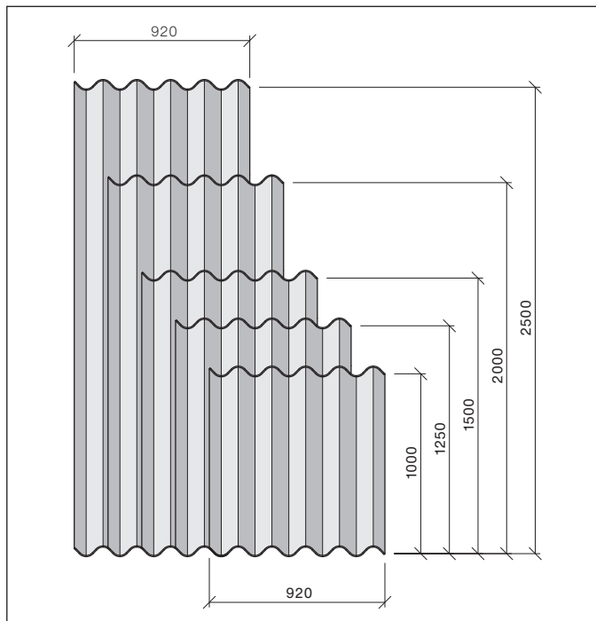
Plaque ondulée Ondapress-57 type 0, sans angle estampé
