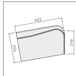
About de faîtière d'appentis 80°
