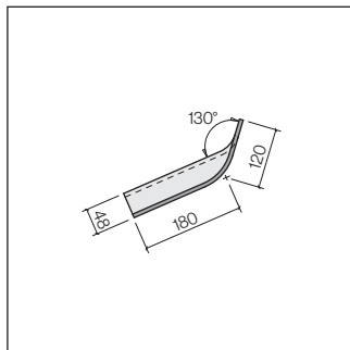
Raccord de faîtière
