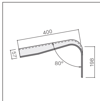
Faîtière d'appentis 80°
