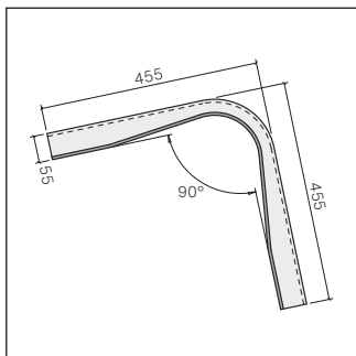
Faîtière angulaire 90°
