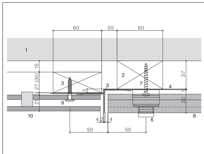
Coupe horizontale, raccord de façade vers Clinker Clip 6 mm
