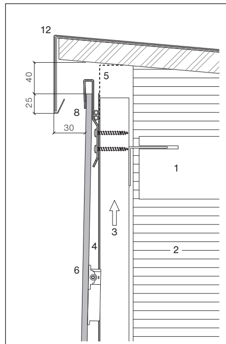
Raccord avec module PV pour appui intermédiaire
