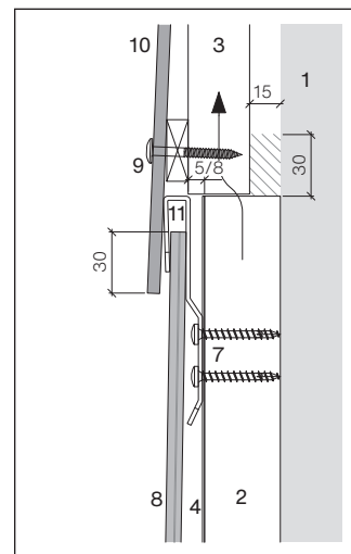
Coupe verticale, raccord de façade vers Clinear Clip 6 mm
