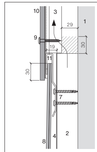
Coupe verticale, raccord de façade vers Largo 8 mm
