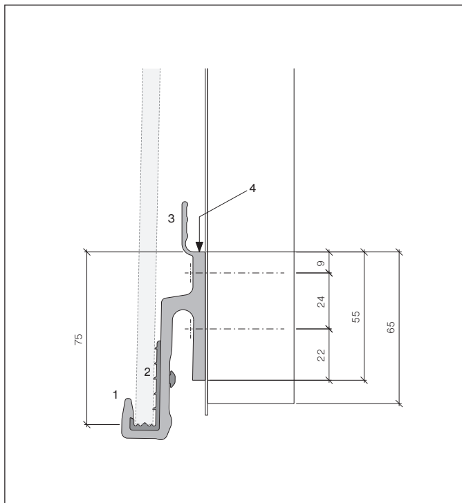
Fixation avec 2 vis, 5.0×40 mm par crochet de module initial
