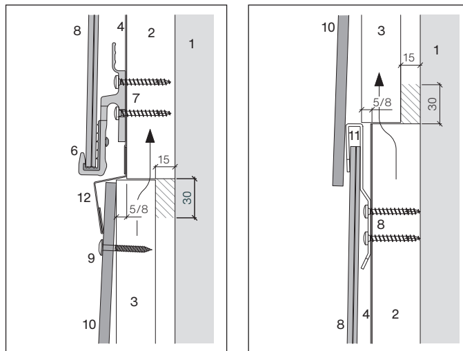
Passage en haut
