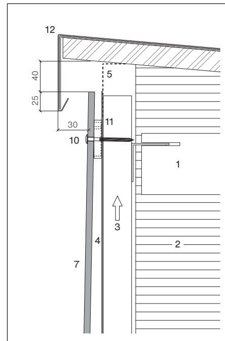
Raccord avec plaques complémentaires, fixé visiblement
