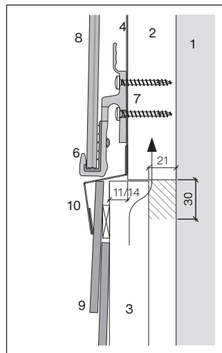
Coupe verticale, raccord de façade vers pose à clin Clinar 6 mm
