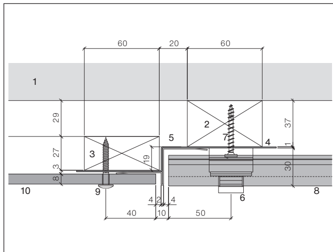
Coupe horizontale, raccord de façade vers Largo 8 mm
