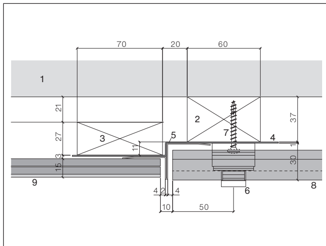
Coupe horizontale, raccord de façade vers pose à clin Clinar 6 mm
