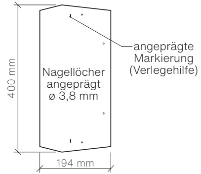
ED Steinschindel 194x385 mm
