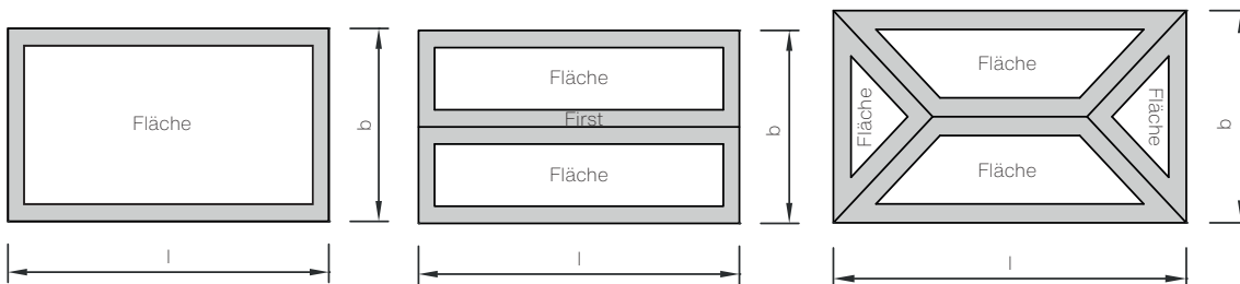
Saumbereich bei Pultdach
